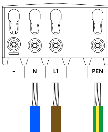
Sieć TN-C-S (PME)
