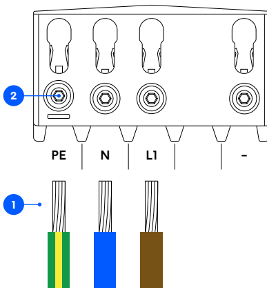
Sieć TT / TN-S
